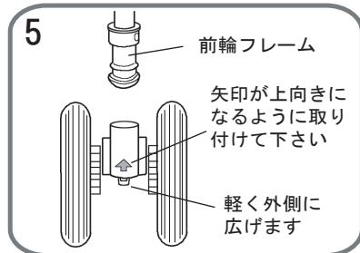
5. 前輪を前輪フレームに取付けてください。 プラスチックのペロを外側に軽く広げて 車輪側の矢印が上向きになるように取付けてください。
